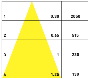
18° UGR<10
