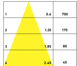
36° UGR<19
