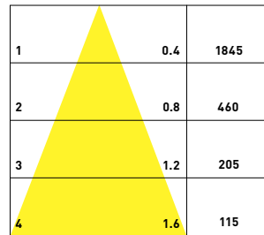
24° UGR<19
