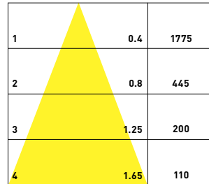
24° UGR<10
