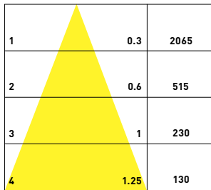
18° UGR<19
