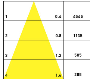
30° UGR<19
