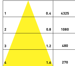
30° UGR<10
