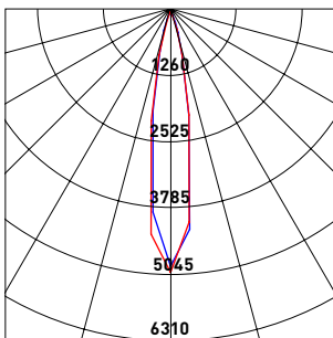
15° UGR<10
