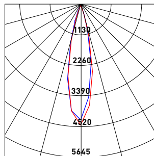
30° UGR<10
