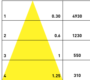
15° UGR<10
