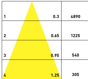
15° UGR<19
