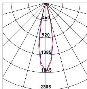
30° UGR<19
