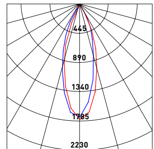
45° UGR<10
