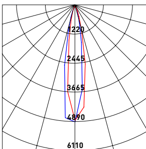
15° UGR<19
