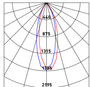
45° UGR<19
