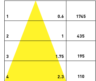
45° UGR<10
