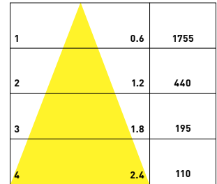
45° UGR<19
